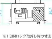
※1 DINロック取外し時の寸法
