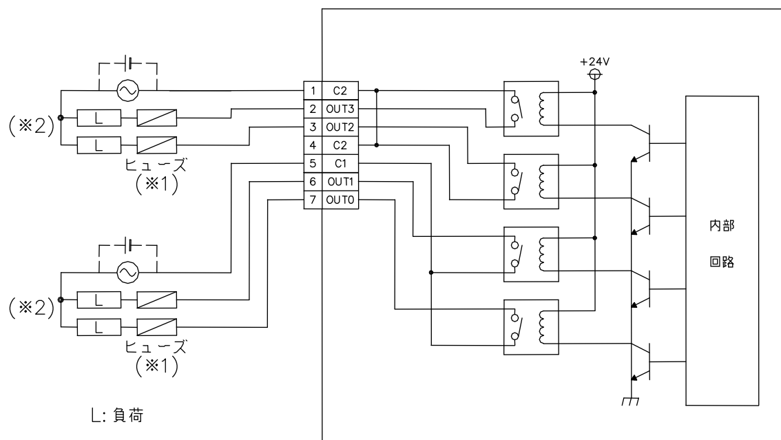
コモン分離接続図(例)
