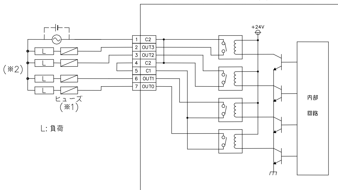
コモン共通接続図(例)
