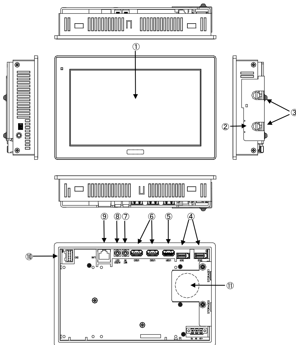
図 3-1-1. 外形図 (APS4-070BN)
