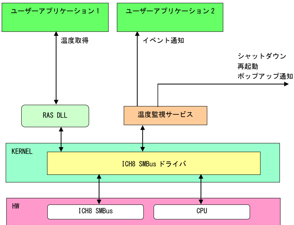
図 5-8-2-1. RAS DLL
