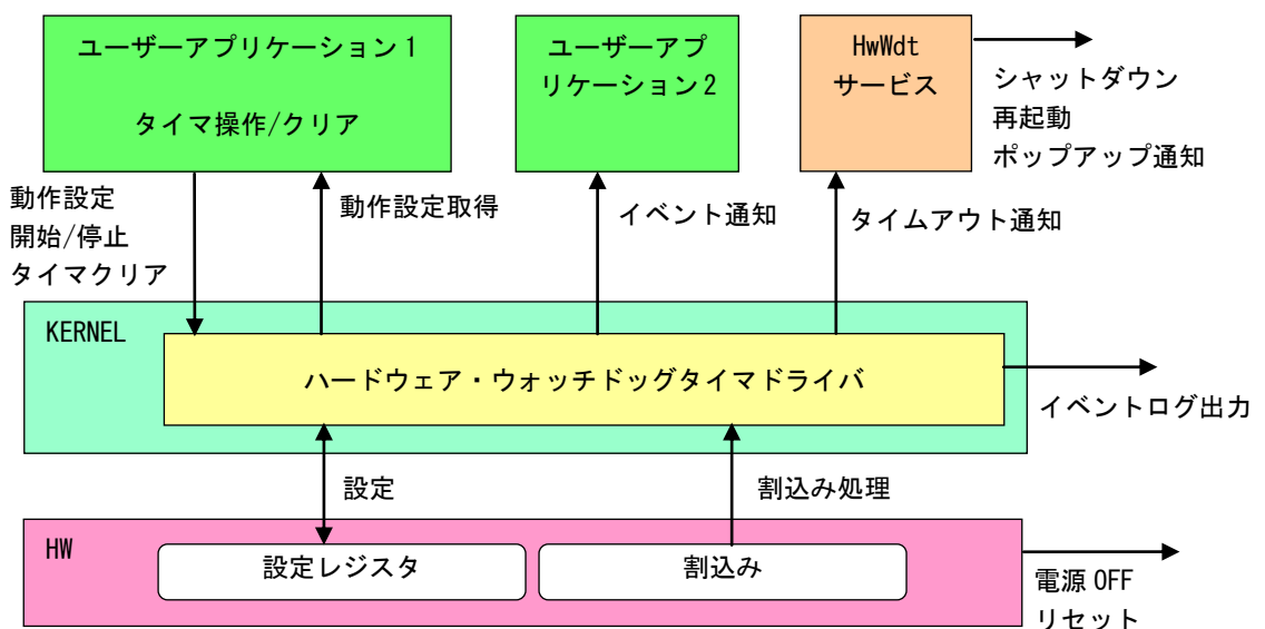
図 5-6-2-1. ハードウェア・ウォッチドッグタイマドライバ
