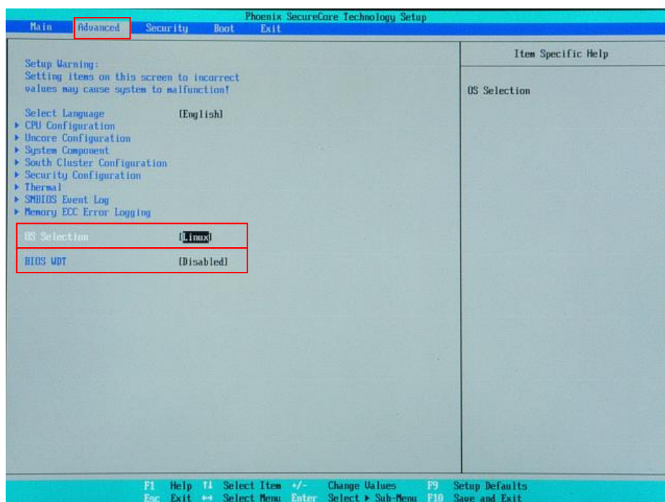
図 6-1-1-1. BIOS 設定 Advanced メニュー
