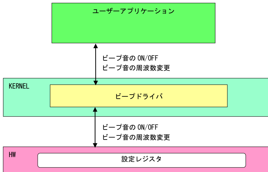
図 5-10-2-1. ビープドライバ
