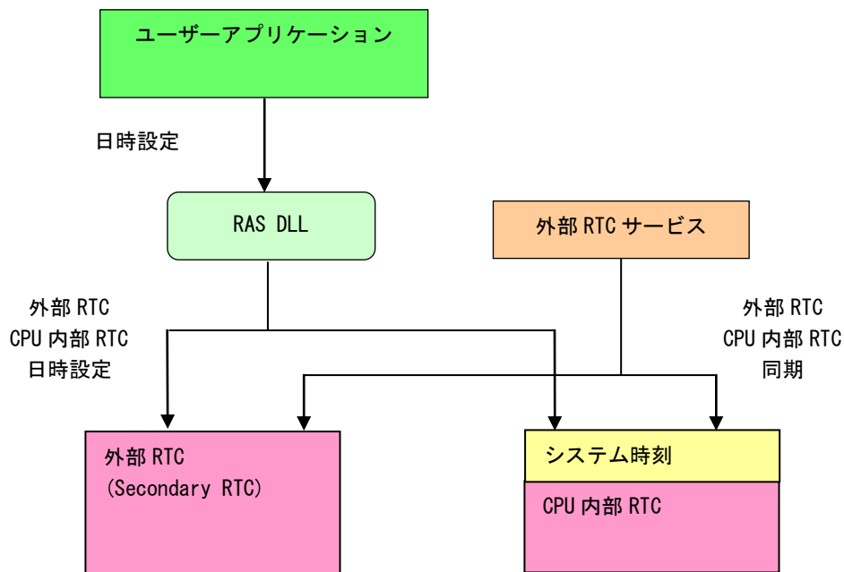
図 5-9-2-1. RAS DLL 日時設定
