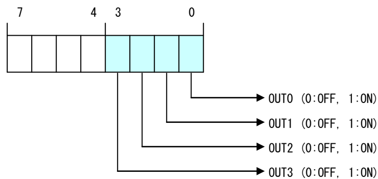
図 5-3-1-2. 出力データ
