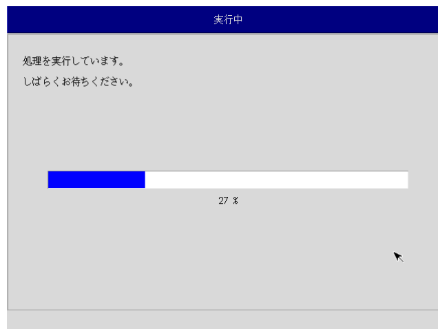
図 6-3-7. 実行中画面
