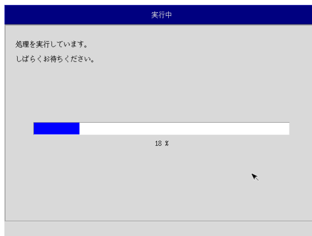
図 6-2-6. 実行中画面
