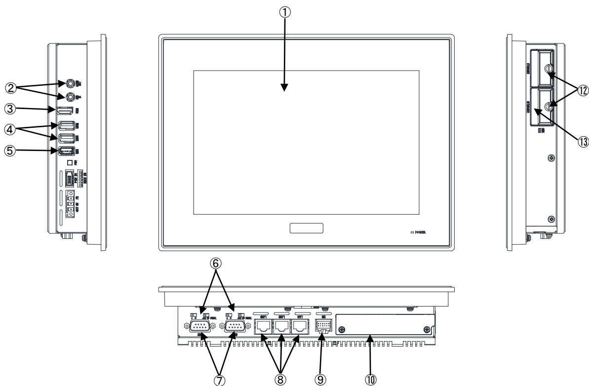
図 3-1-1. 外形図 (AP4A-101AN)
