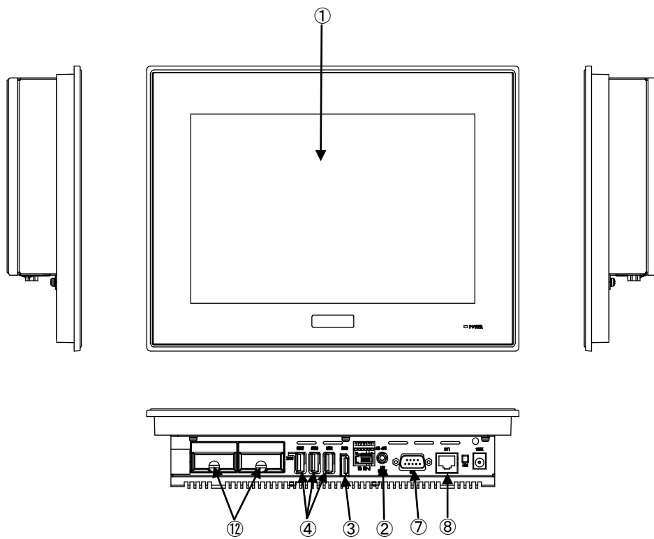
図 3-1-3. 外形図 (APL4A-101BN)
