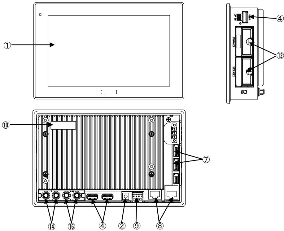
図 3-1-7. 外形図 (APS4A-070DN/DS)
