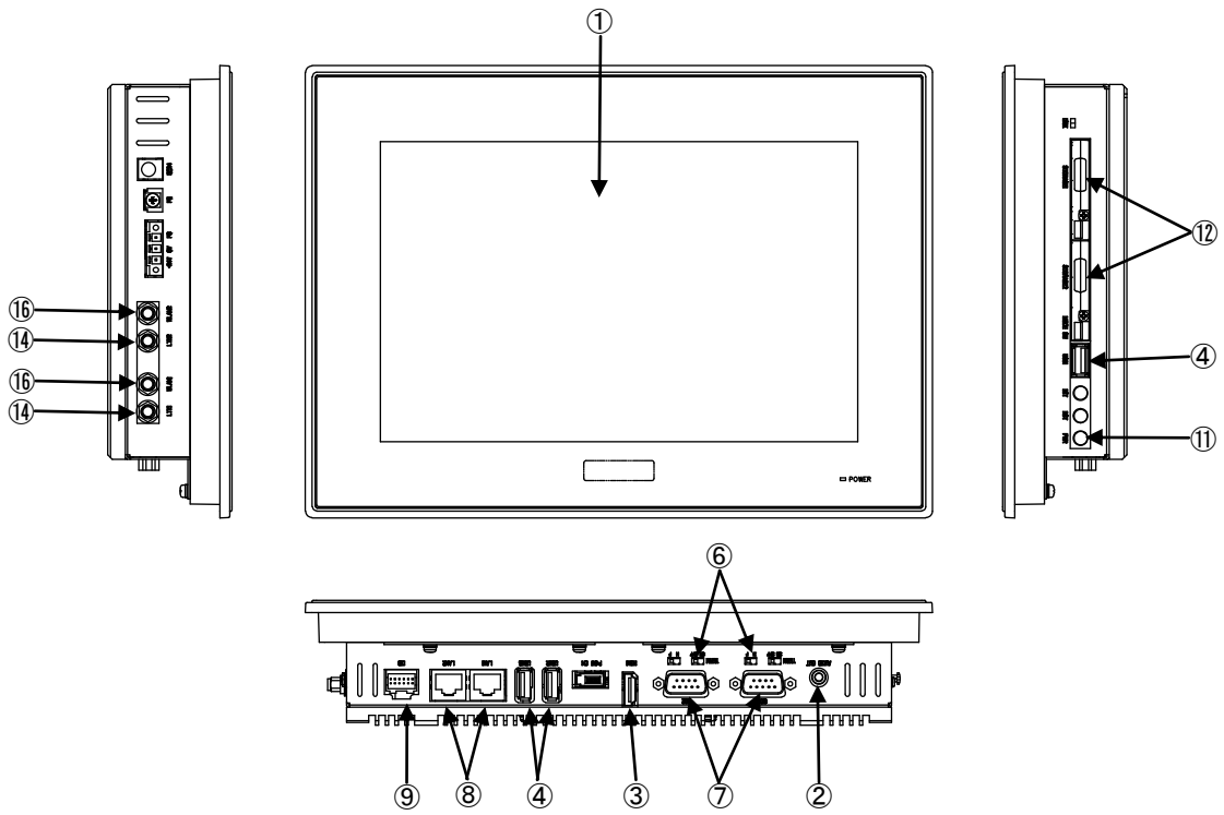
図 3-1-6. 外形図 (APS4A-101DN)
