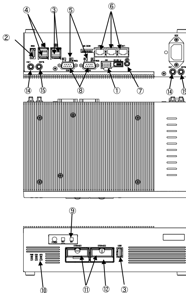
図 3-1-3. 外形図 (EC4A-100CA)
