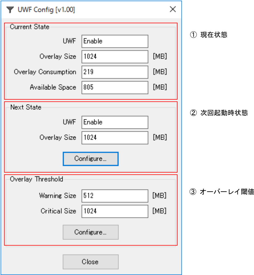
図 2-3-4-4. UWF Config Tool 設定画面
