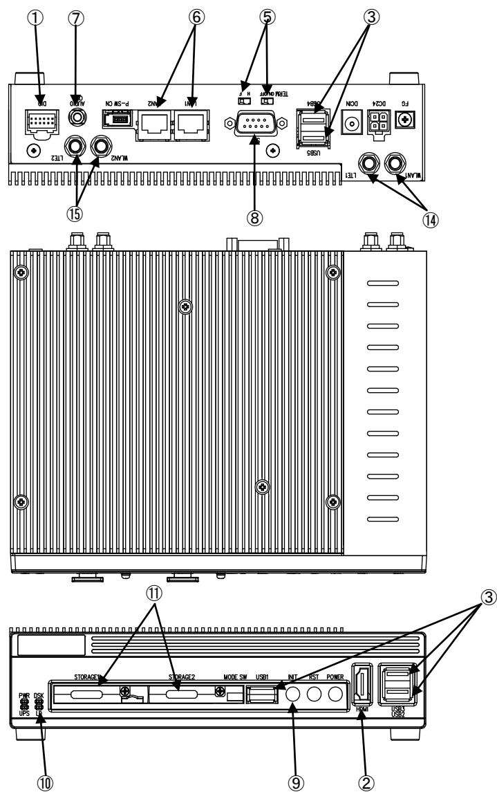
図 3-1-2. 外形図 (EC4A-010CT)
