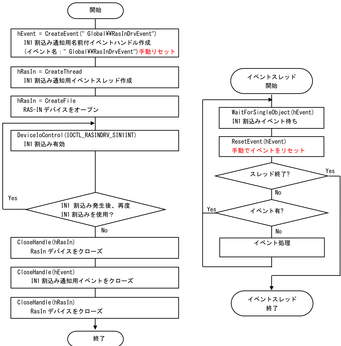
図 4-4-5-1. 複数アプリケーションで IN1 割り込みを使用する手順
