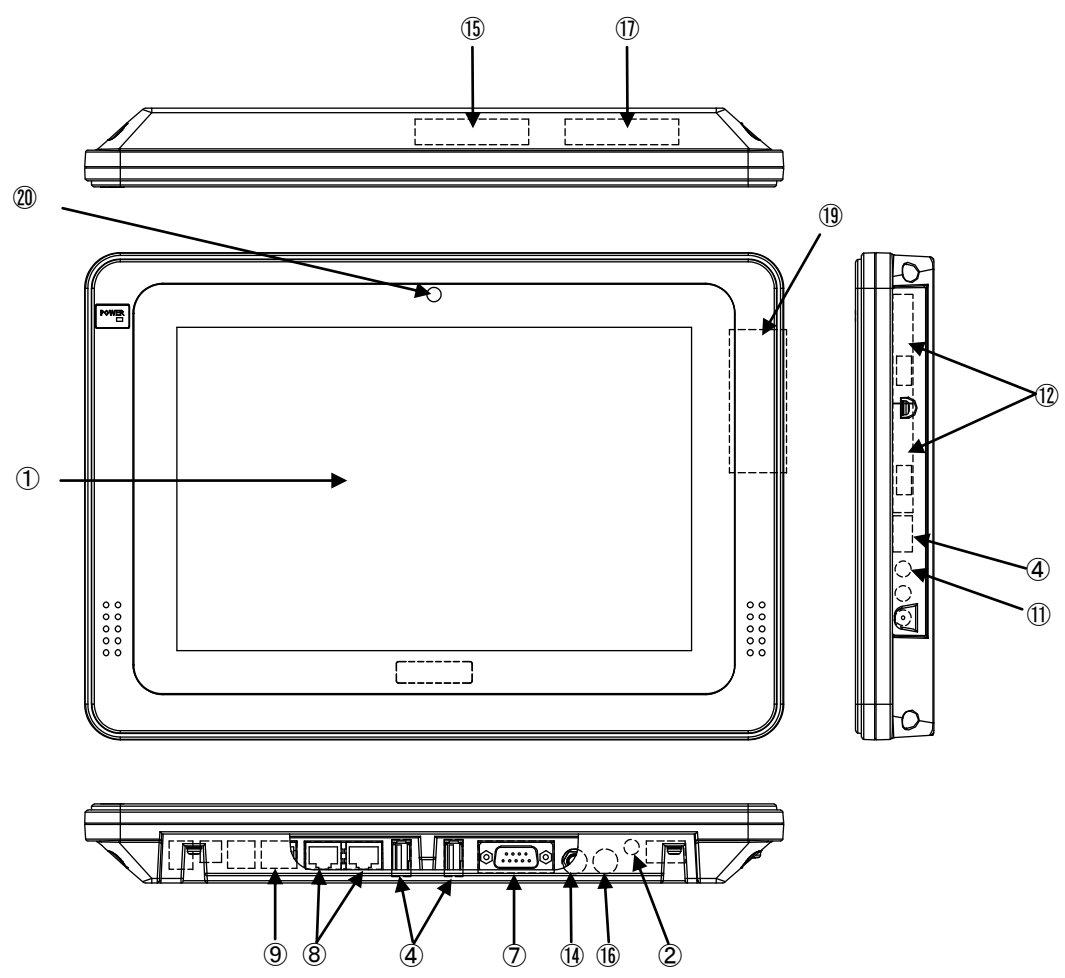
図 3-1-8. 外形図 (AS4A-101DN/DS)
