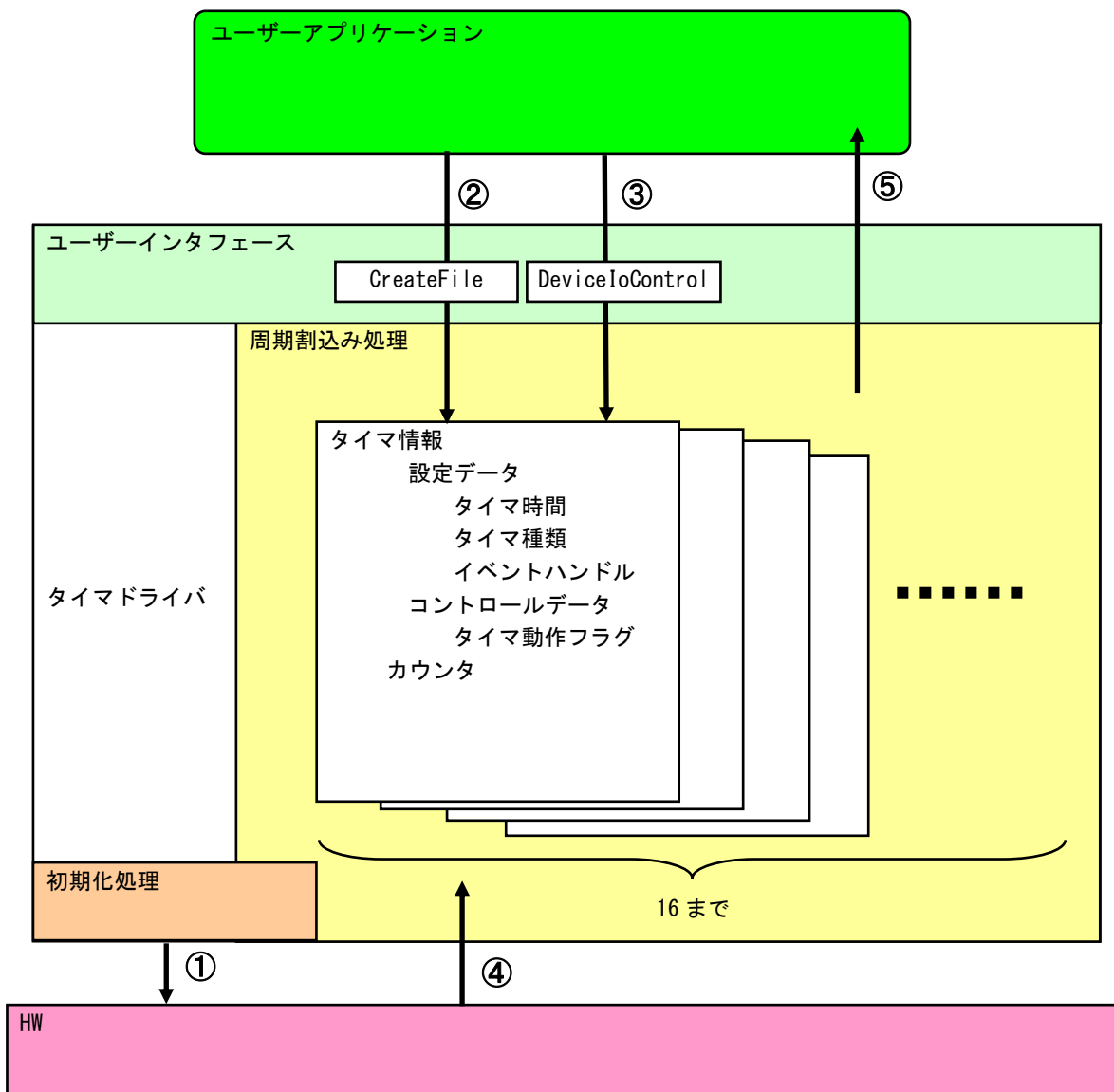
図 5-2-4-1. タイムドライバの動作
