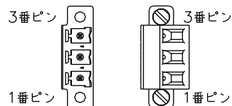
ケーブル側コネクタ図
