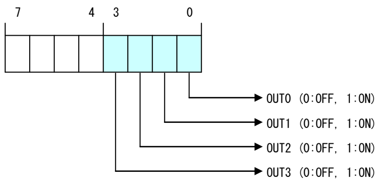
図 4-3-1-2. 出力データ
