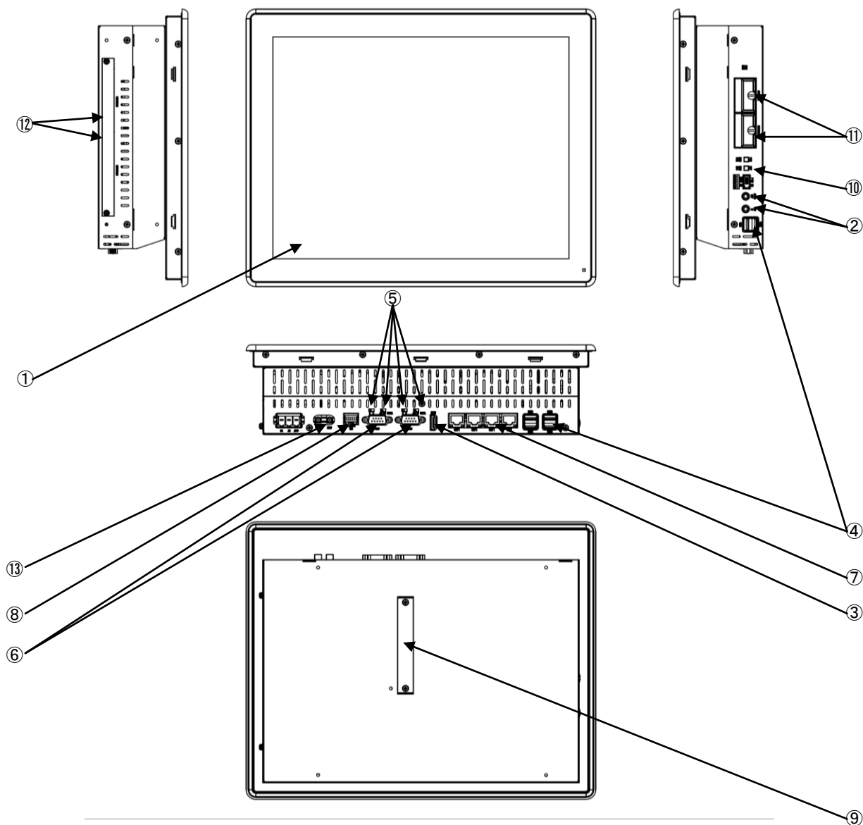
図 3-1-1. 外形図 (AP7A-150AN)
