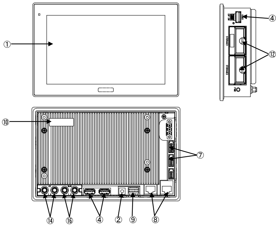
図 3-1-3. 外形図 (APS4B-070BN/BS)
