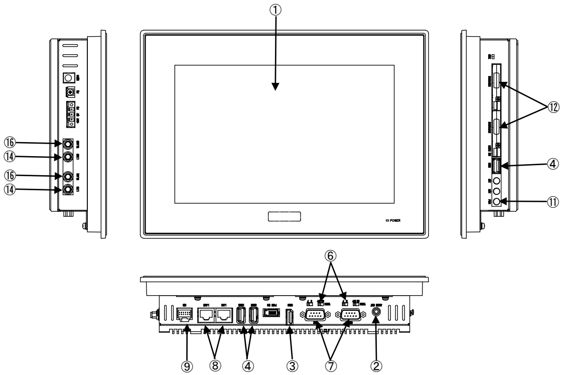
図 3-1-2. 外形図 (APS4B-101BN)
