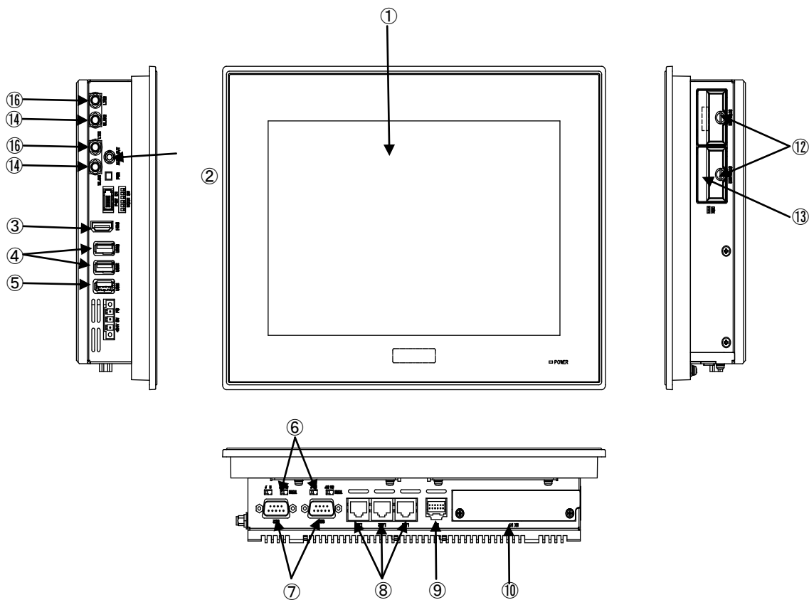
図 3-1-1. 外形図 (AP4B-101AN)
