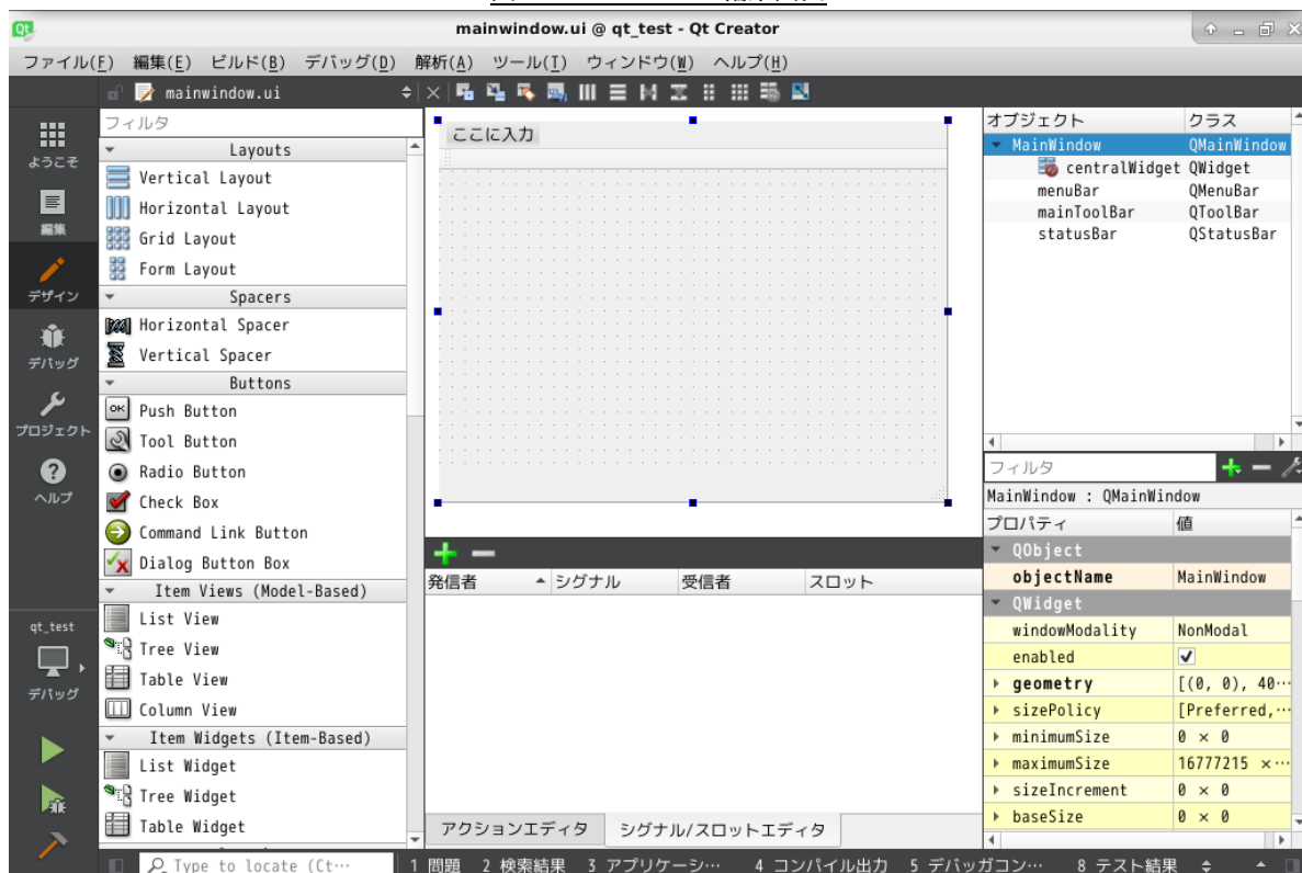
図 2-4-4-8. フォーム画面編集画面
