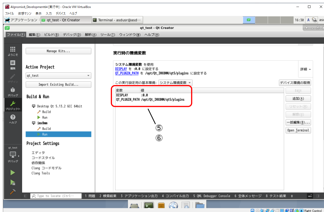
図 2-4-9-9. 実行時の環境変数設定（DISPLAY 環境変数設定）
